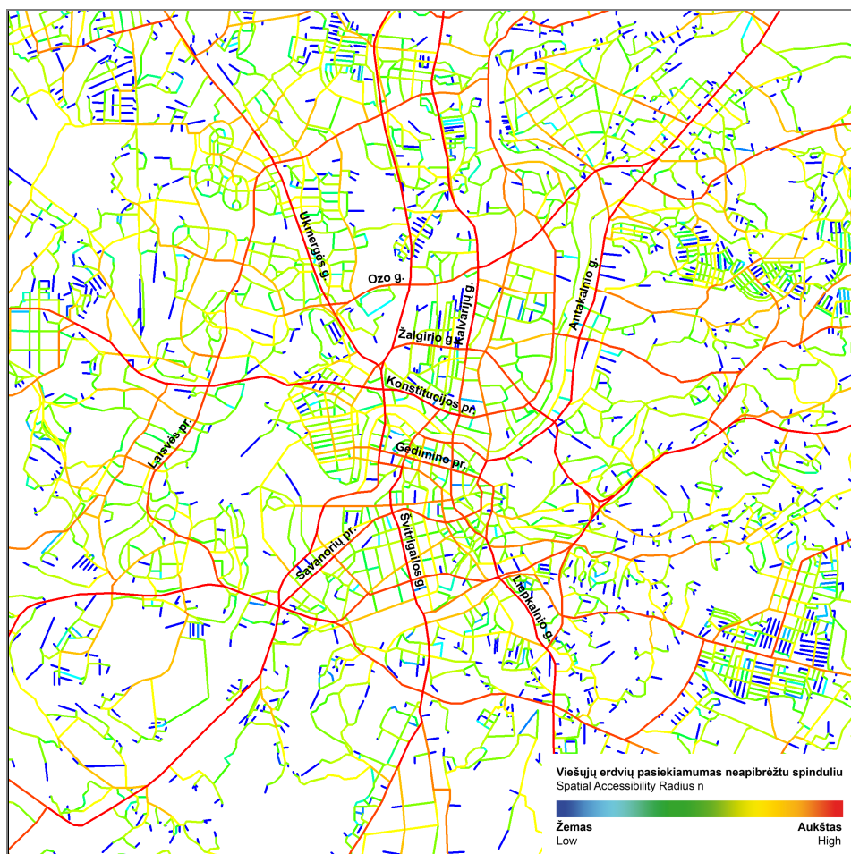
A4 pav. Vilniaus miesto viešųjų erdvių pasiekiamumo neapibrėžtu spinduliu schema ( through-movement ; pasirinkimas, įvertinant mažiausią posūkio kampą)
