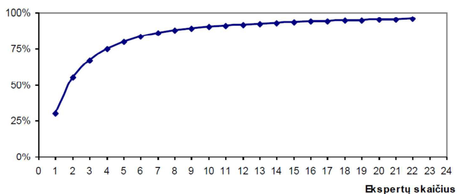
G.1 pav. Ekspertų vertinimų standartinio nuokrypio priklausomybė nuo ekspertų skaičiaus (šaltinis: Urbonienė, 2014)
