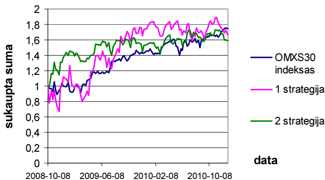
J.2 pav. OMXS30 indekso (Švedija) ir dviejų sistemos strategijų palyginimas. Portfelio rebalansavimas atliekamas su savaitės trukmės duomenimis pagal pirmos savaitės dienos akcijų kainas
