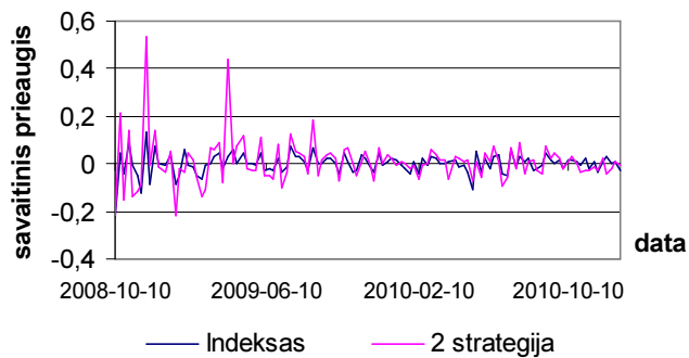
I.4 pav. Kas savaitę fiksuojami CAC 40 indekso ir lėšų sumos, investuotos pagal 2-ą strategiją, prieaugiai
