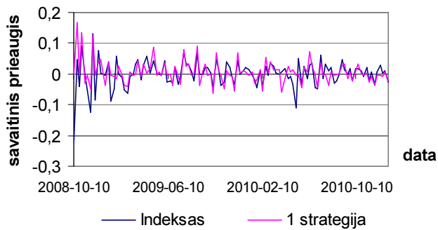
I.3 pav. Kas savaitę fiksuojami CAC 40 indekso ir lėšų sumos, investuotos pagal 1-ą strategiją, prieaugiai
