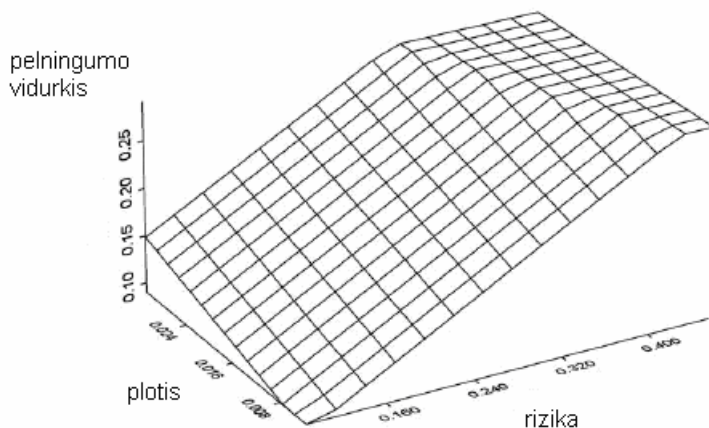
A.1 pav. Pelningumo, rizikos ir pločio portfelio trimatis vaizdas
