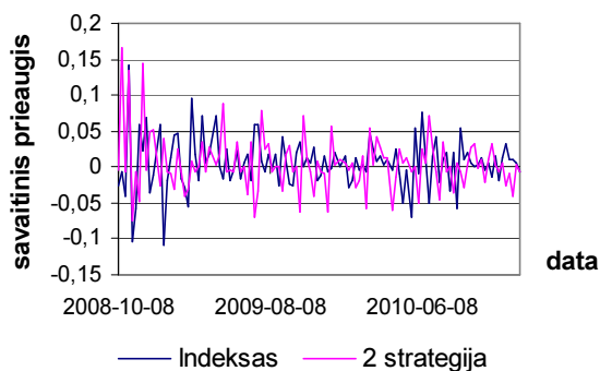
J.4 pav. Kas savaitę fiksuojami OMXS30 indekso ir lėšų sumos, investuotos pagal 2-ą strategiją, prieaugiai
