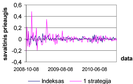
J.3 pav. Kas savaitę fiksuojami OMXS30 indekso ir lėšų sumos, investuotos pagal 1-ą strategiją, prieaugiai
