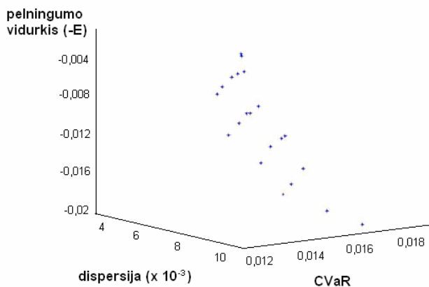
A.2 pav. Efektyvusis portfelio paviršius vidurkio – dispersijos – CVaR erdvėje
