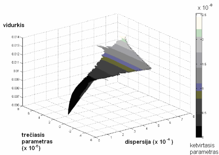
A.3 pav. Vidurkio – dispersijos – asimetrijos – eksceso efektyvusis paviršius vidurkio – dispersijos – trečiojo parametro erdvėje (skirtingo pilkumo atspalviai žymi ketvirtojo parametro – eksceso lygį)
