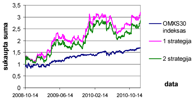
J.1 pav. OMXS30 indekso (Švedija) ir dviejų sistemos strategijų palyginimas. Portfelio rebalansavimas atliekamas pagal dienos trukmės akcijų kainas
