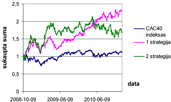
I.1 pav. CAC 40 indekso (Prancūzija) ir dviejų sistemos strategijų palyginimas. Portfelio rebalansavimas atliekamas pagal dienos trukmės akcijų kainas
