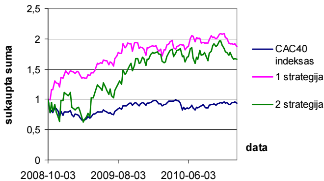
I.2 pav. CAC 40 indekso (Prancūzija) ir dviejų sistemos strategijų palyginimas. Portfelio rebalansavimas atliekamas su savaitės trukmės duomenimis pagal pirmos savaitės dienos akcijų kainas
