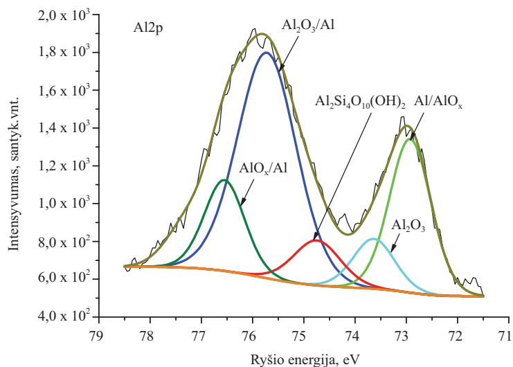
D6 pav. Aliuminio Al 2 p smailės rentgeno fotoelektronų spektras nuvalius aliuminio-magnio lydinio paviršių \text{Al}_2\text{O}_3 srautu ir fosforo rūgšties tirpalu Fig. D6. X-ray photoelectron spectrum of aluminium Al 2 p peak after processing the aluminium-magnesium alloy surface by \text{Al}_2\text{O}_3 flow and phosphoric acid solution
