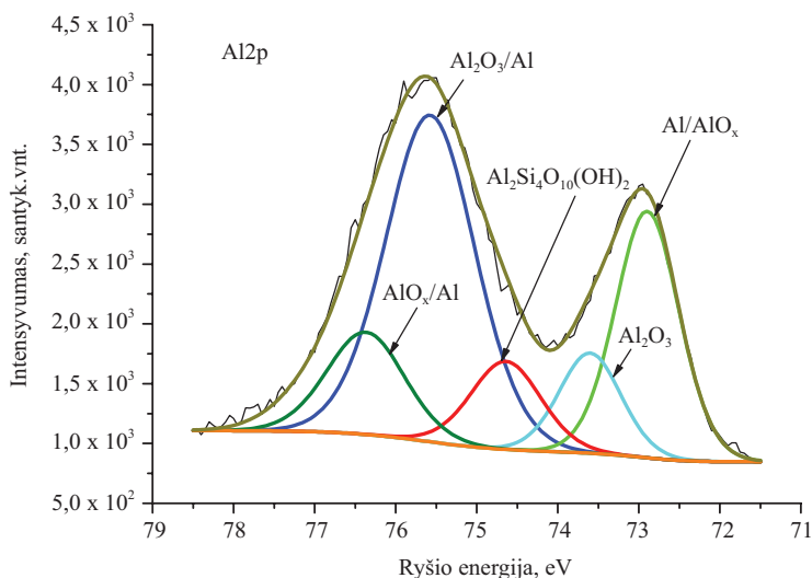
D5 pav. Aliuminio Al 2 p smailės rentgeno fotoelektronų spektras nuvalius aliuminio-magnio lydinio paviršių \text{Al}_2\text{O}_3 srautu ir natrio šarmo, azoto rūgšties tirpalais Fig. D5. X-ray photoelectron spectrum of aluminium Al 2 p peak after processing the aluminium-magnesium alloy surface by \text{Al}_2\text{O}_3 flow and sodium hydroxide & nitric acid solutions
