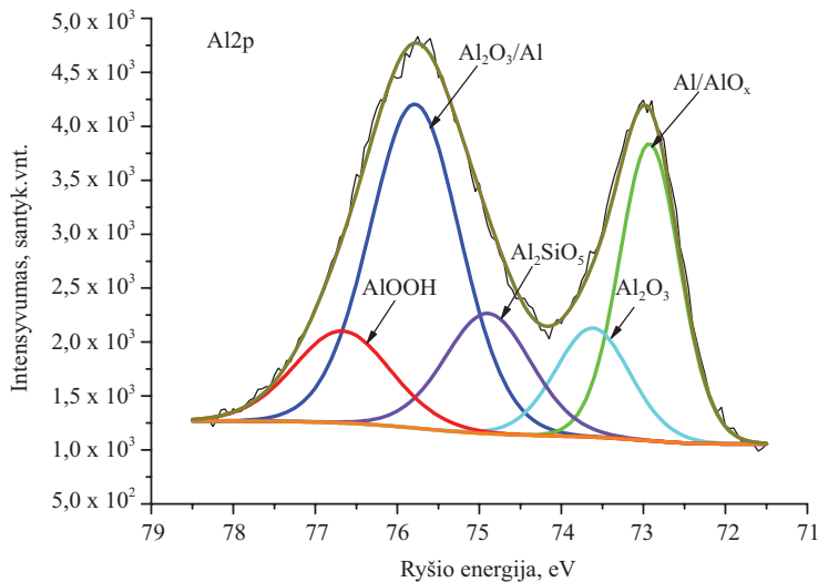
D3 pav. Aliuminio Al 2 p smailės rentgeno fotoelektronų spektras nuvalius aliuminio-magnio lydinio paviršių fosforo, azoto rūgščių ir vario sulfato tirpalu Fig. D3. X-ray photoelectron spectrum of aluminium Al 2 p peak after processing the aluminium-magnesium alloy surface by phosphoric acid, nitric acid and copper sulphate solution
