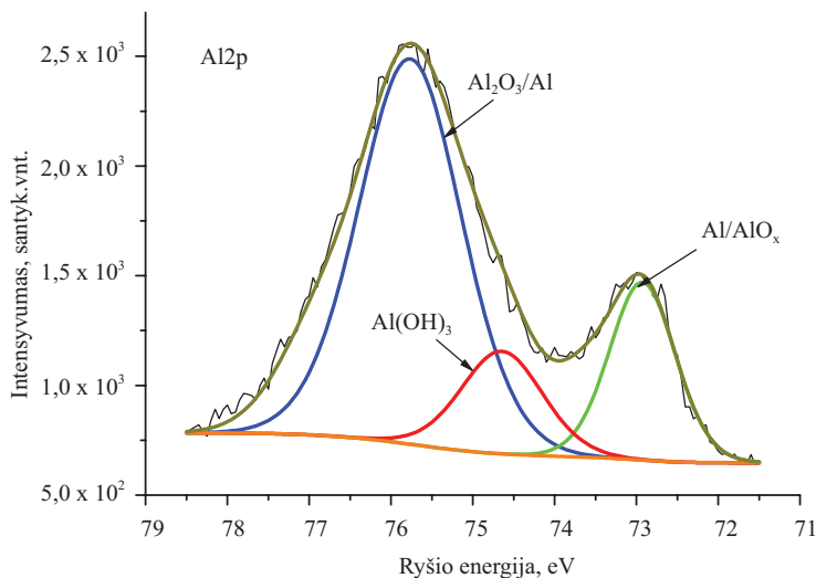
D4 pav. Aliuminio Al 2 p smailės rentgeno fotoelektronų spektras nuvalius aliuminio-magnio lydinio paviršių \text{Al}_2\text{O}_3 srautu Fig. D4. X-ray photoelectron spectrum of aluminium Al 2 p peak after processing the aluminium-magnesium alloy surface by \text{Al}_2\text{O}_3 flow
