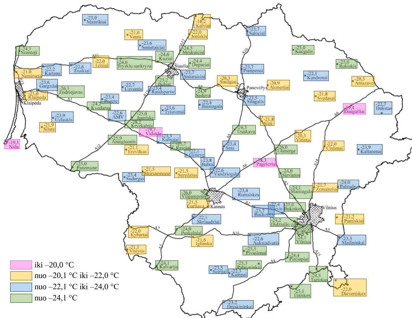
F.1 pav. Žemiausios asfalto dangos paviršiaus temperatūros, užfiksuotos KOS stotelėse 2003–2018 m. Fig. F.1 pav. The lowest surface temperatures of asphalt pavements recorded in road weather stations in 2003–2018
