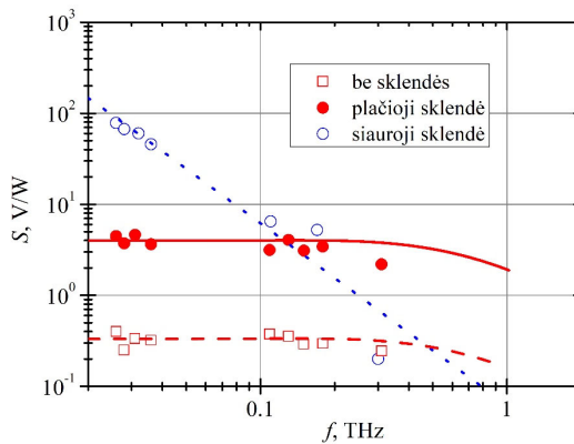
S4.2 pav. Peteliškės formos mikrobangų diodų su dvimačiu elektronų dujų sluoksniu selektyviai legiruotame GaAs/AlGaAs darinyje voltvatinio jautrio dažninės priklausomybės, kai diodas yra be dalinės sklendės ir kai diodo aktyvioji sritis yra uždengta daline sklende plačiojoje arba siaurojoje vietoje
