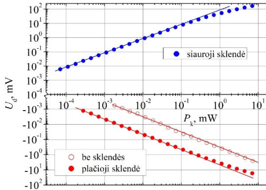
S4.1 pav. Peteliškės formos mikrobangų diodų su dvimačiu elektronų dujų sluoksniu selektyviai legiruotame GaAs/AlGaAs darinyje detektuotos įtampos priklausomybės nuo mikrobangų signalo galios 30 GHz dažnyje, kai diodas yra be dalinės sklendės ir kai diodo aktyvioji sritis yra uždengta su dalinėmis sklendėmis plačiojoje arba siaurojoje diodo aktyviosios srities vietoje
